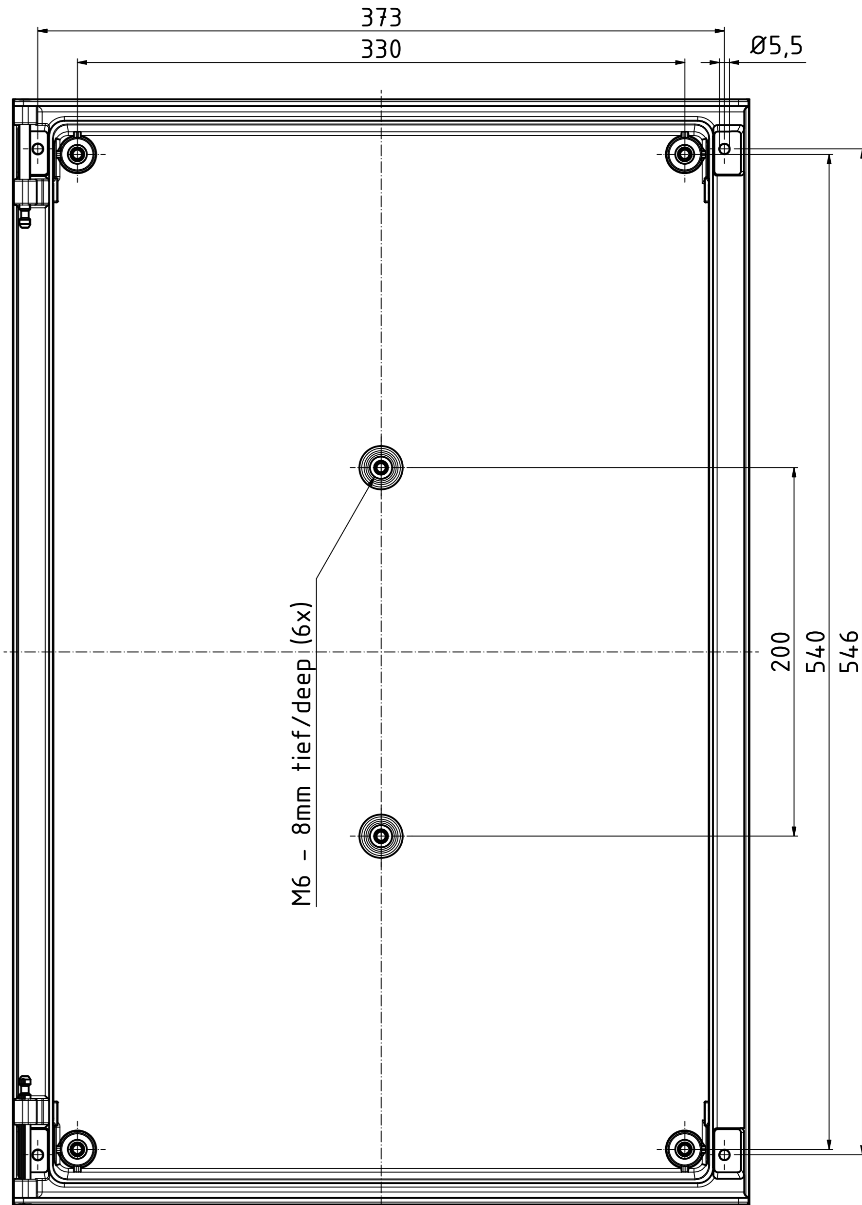
Unterteil ( 1 : 2 ) Base
