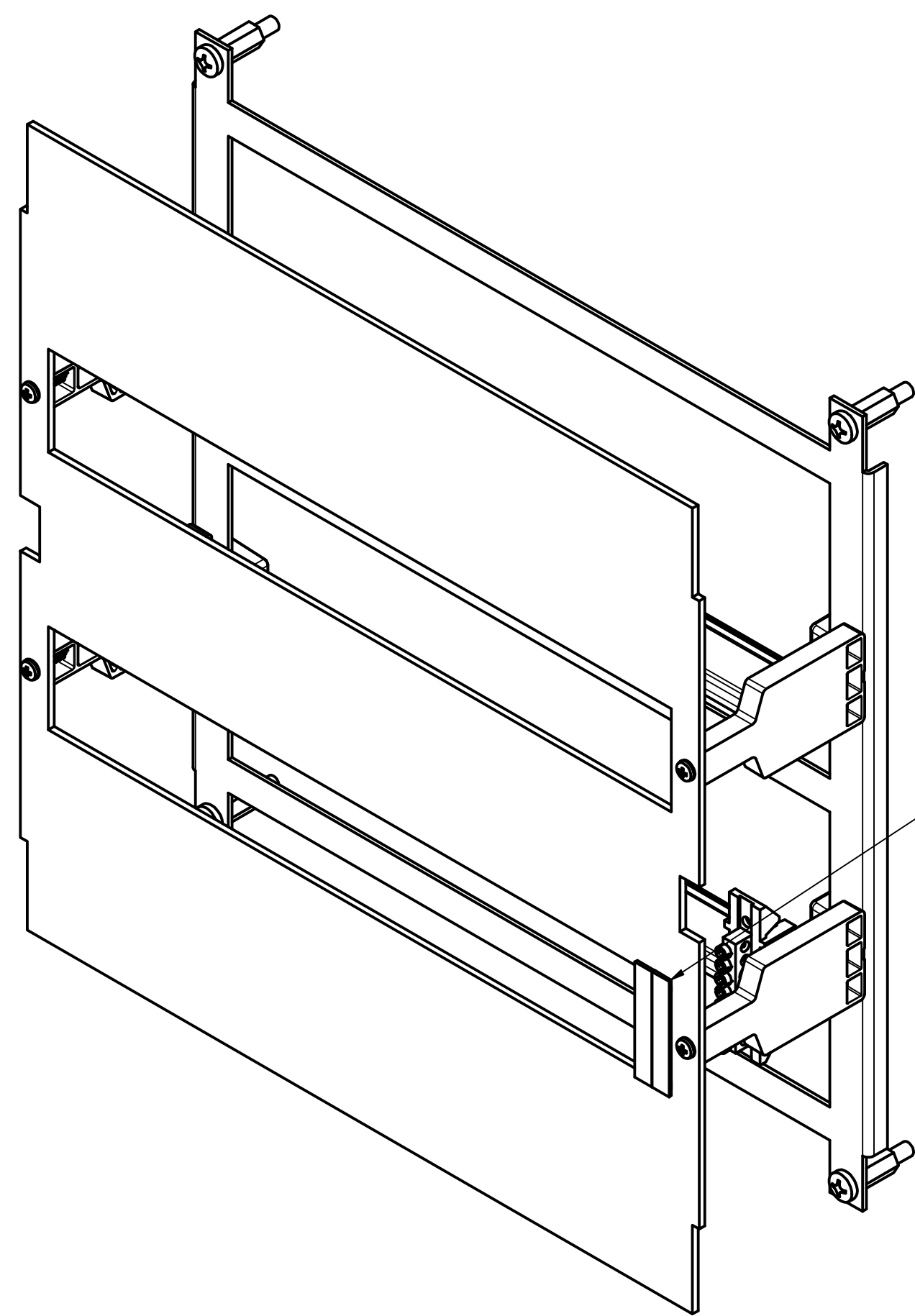
Komplettes Gestell mit Zubehör Complete rack with accessories
