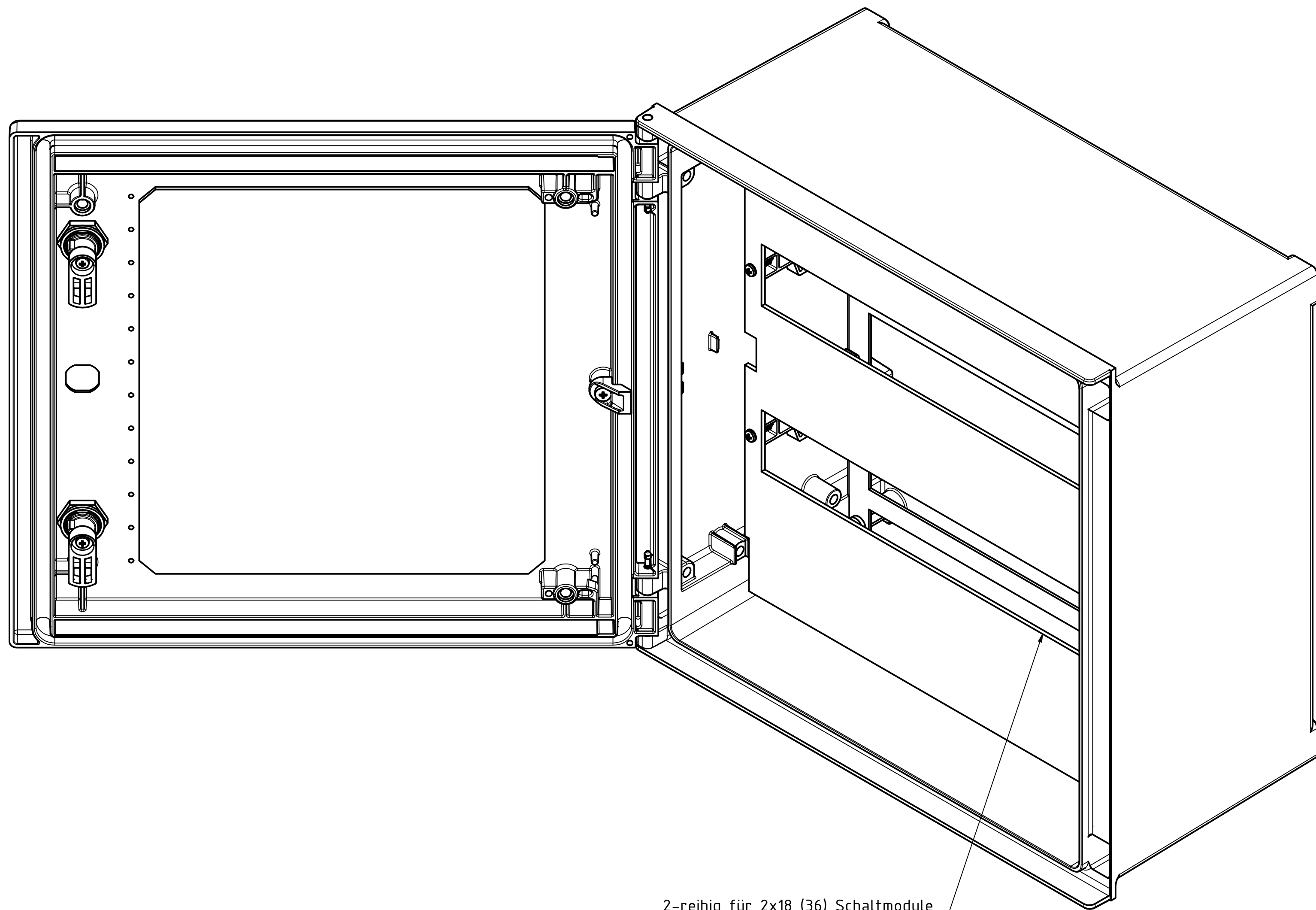
Ansicht ohne Oberteil View without upper part
