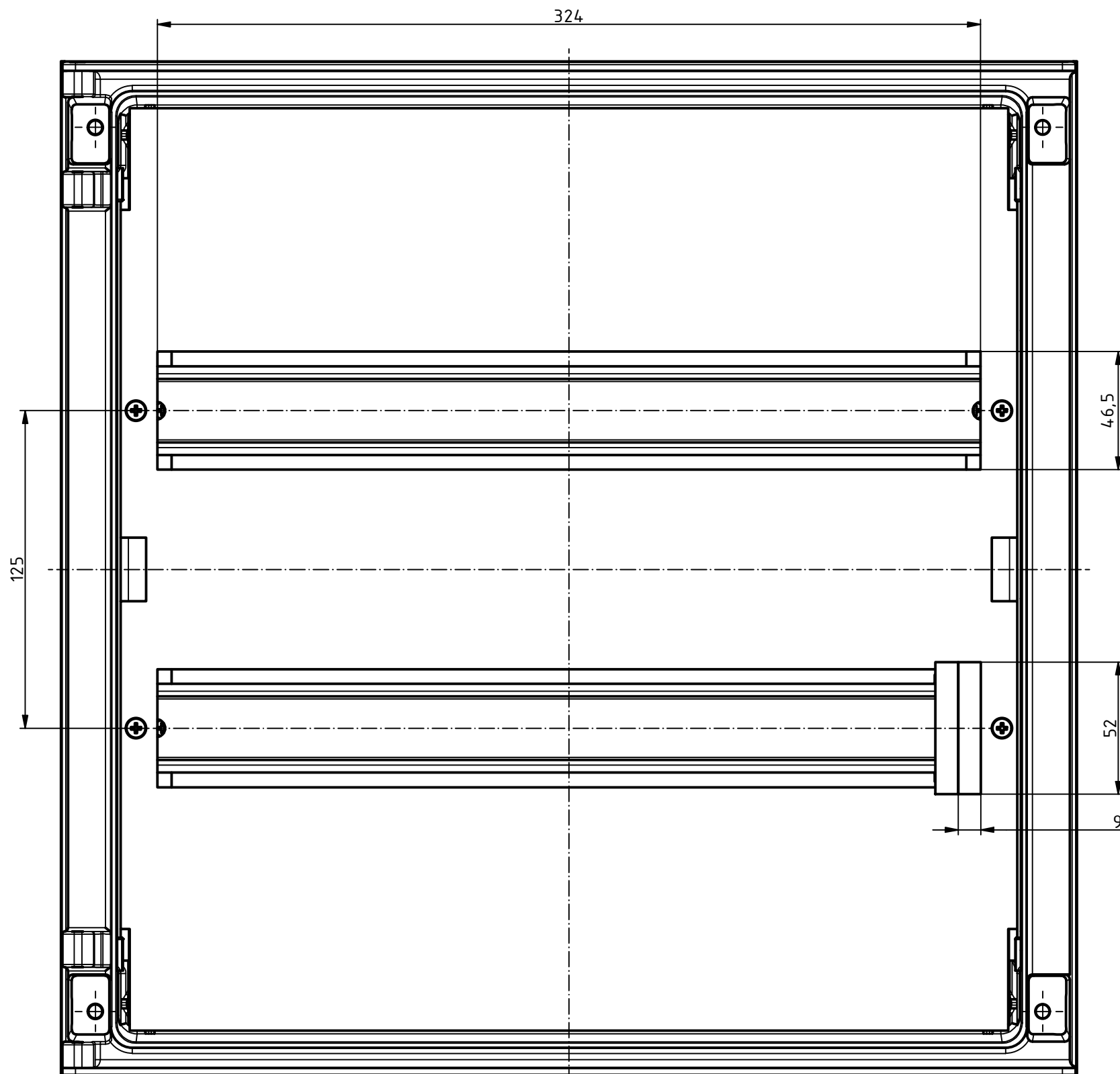
Ansicht ohne Oberteil View without upper part
