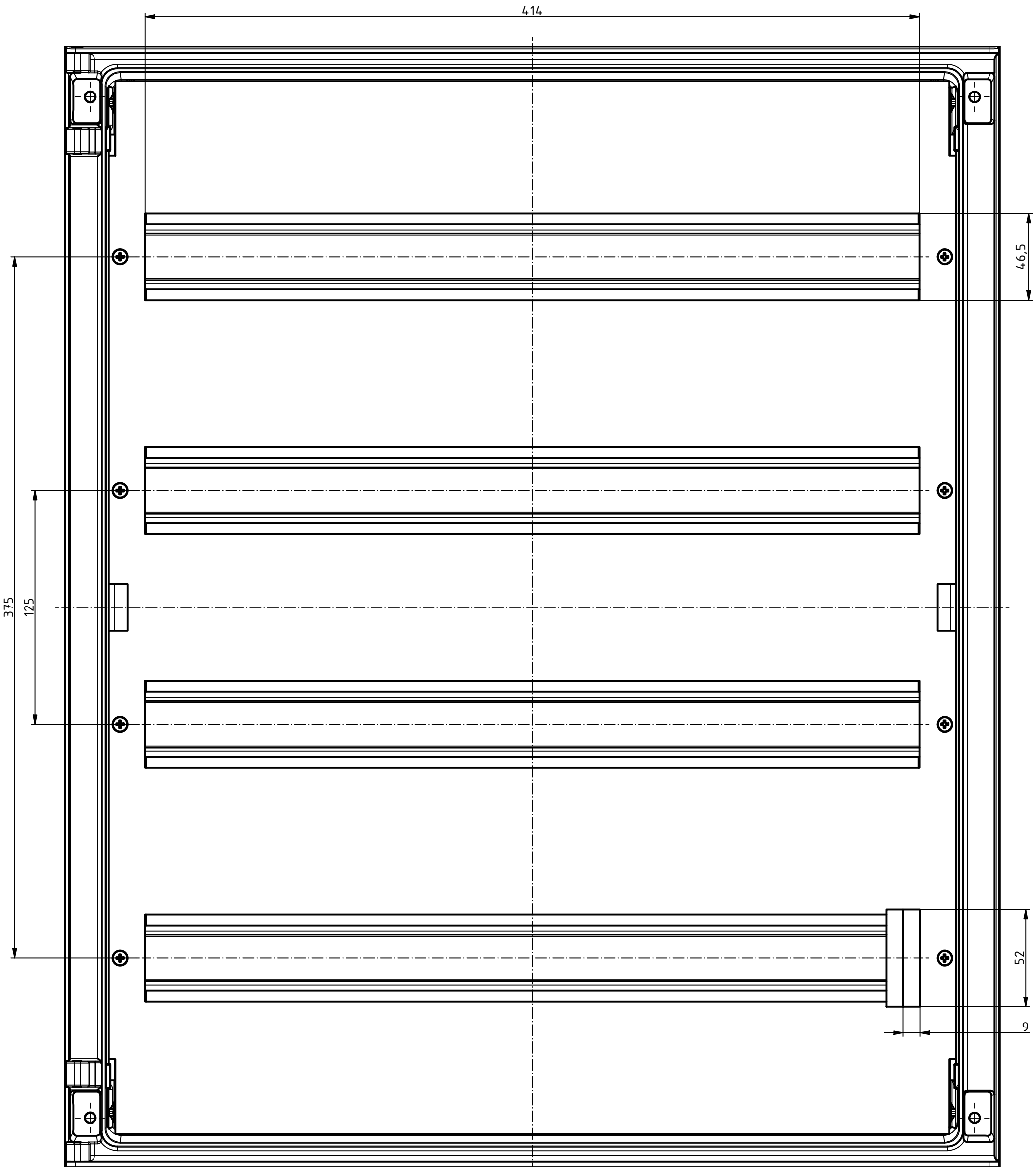
Ansicht ohne Oberteil View without upper part
