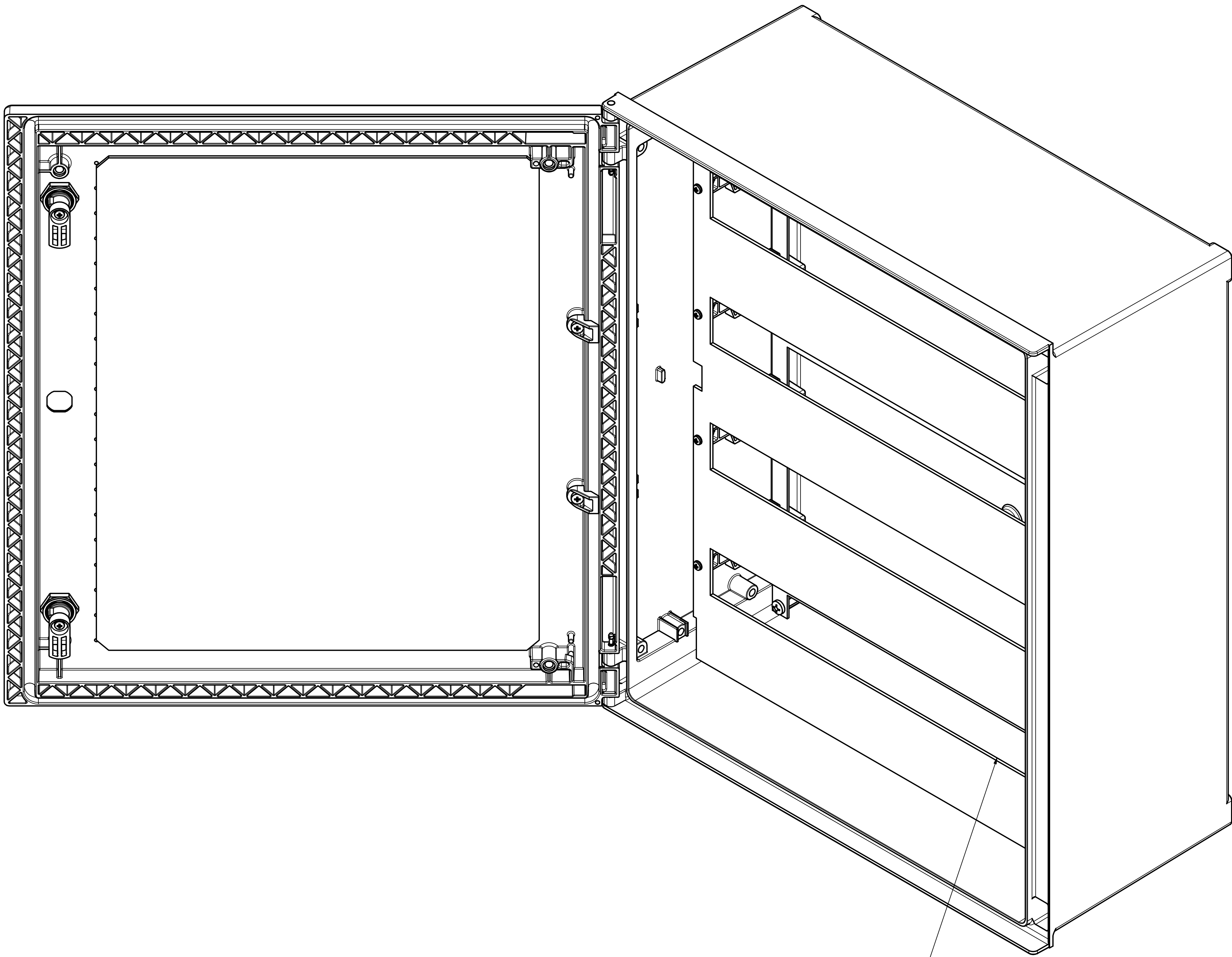
Ansicht ohne Oberteil View without upper part
