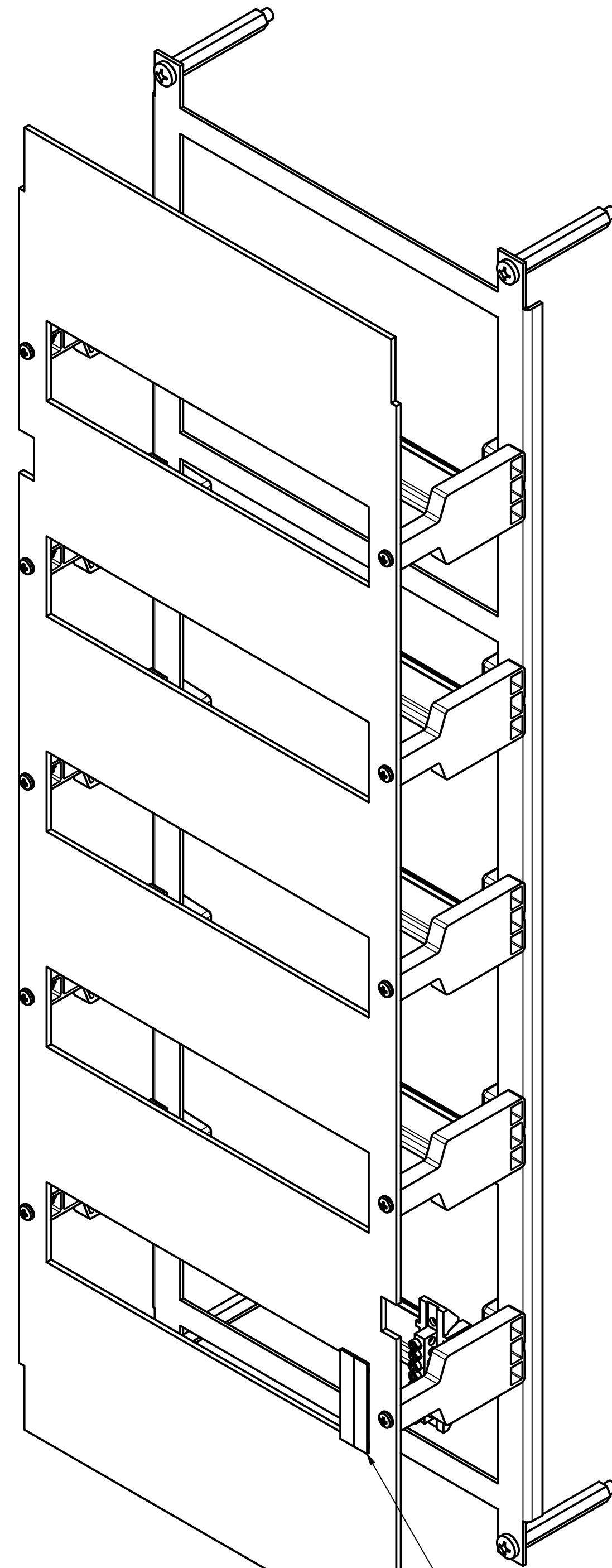
Komplettes Gestell mit Zubehör Complete rack with accessories
