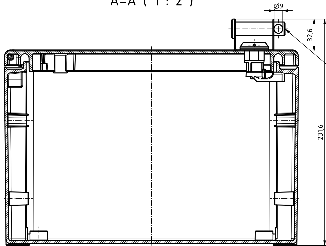
A-A ( 1 : 2 )
