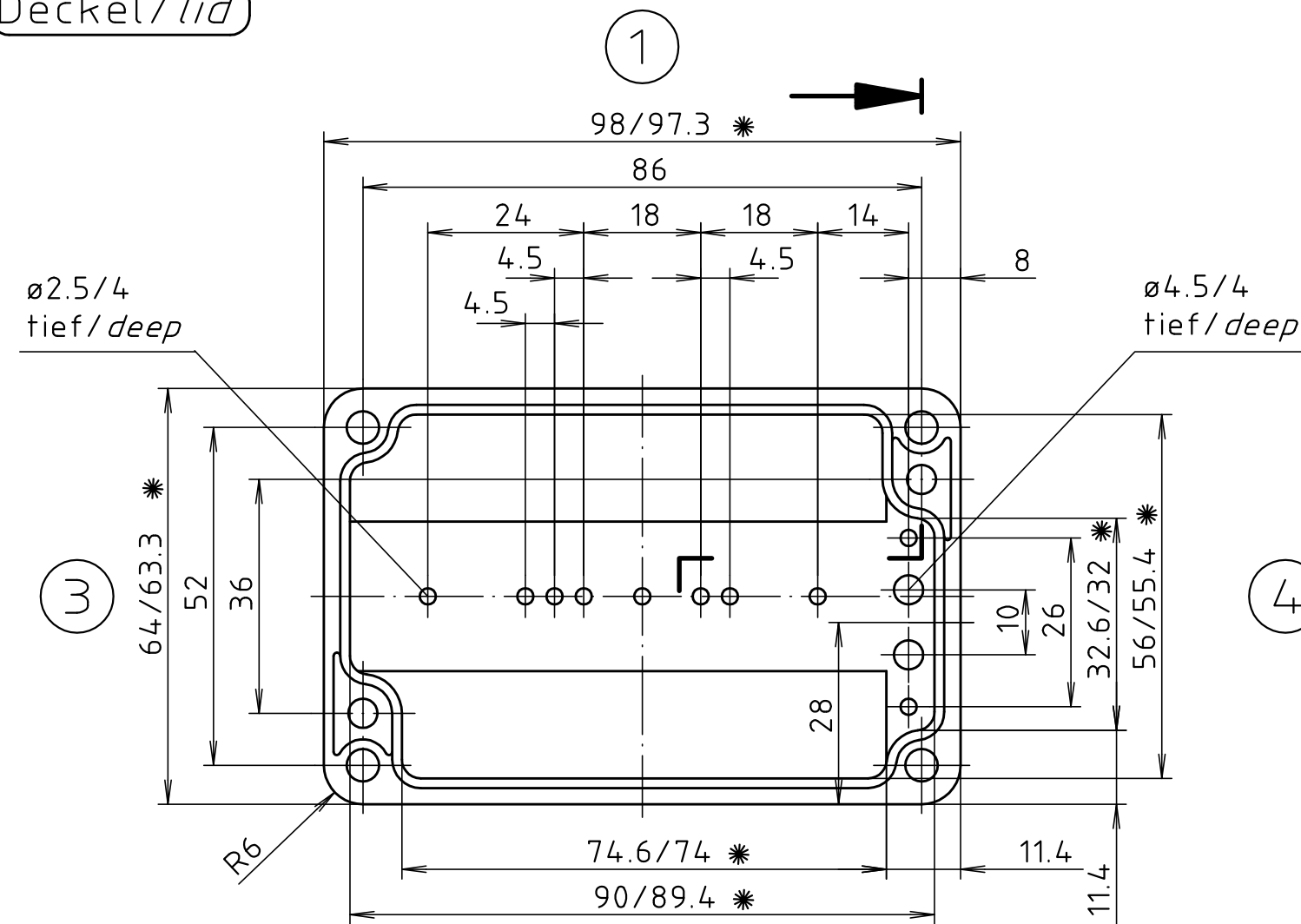
Deckel / lid
