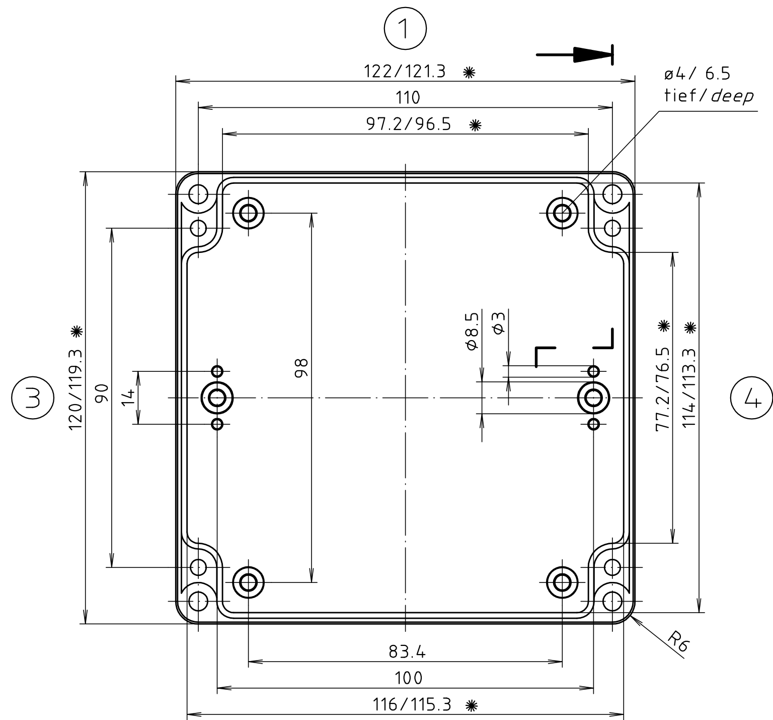
Unterteil / base
