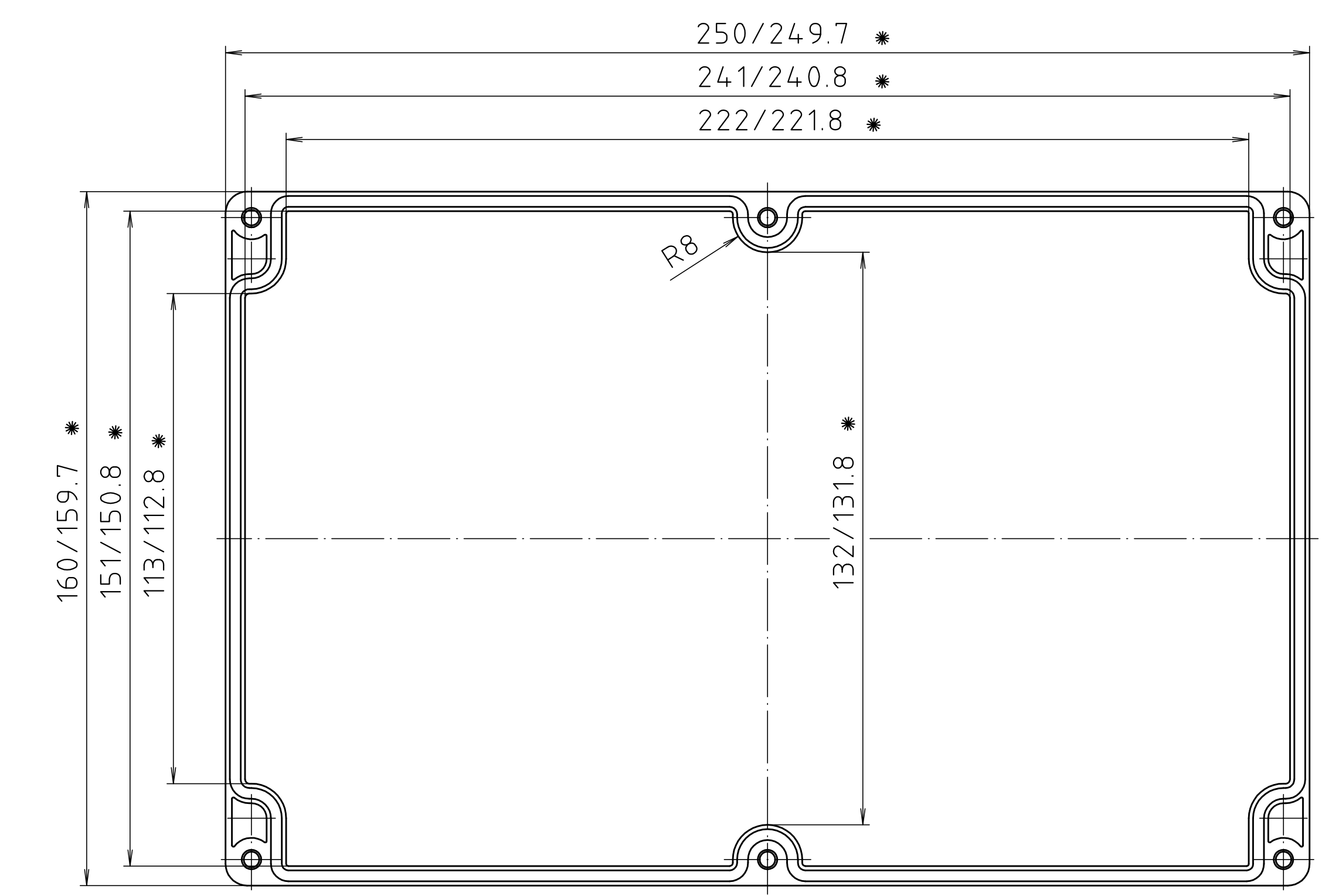
Deckel / lid
