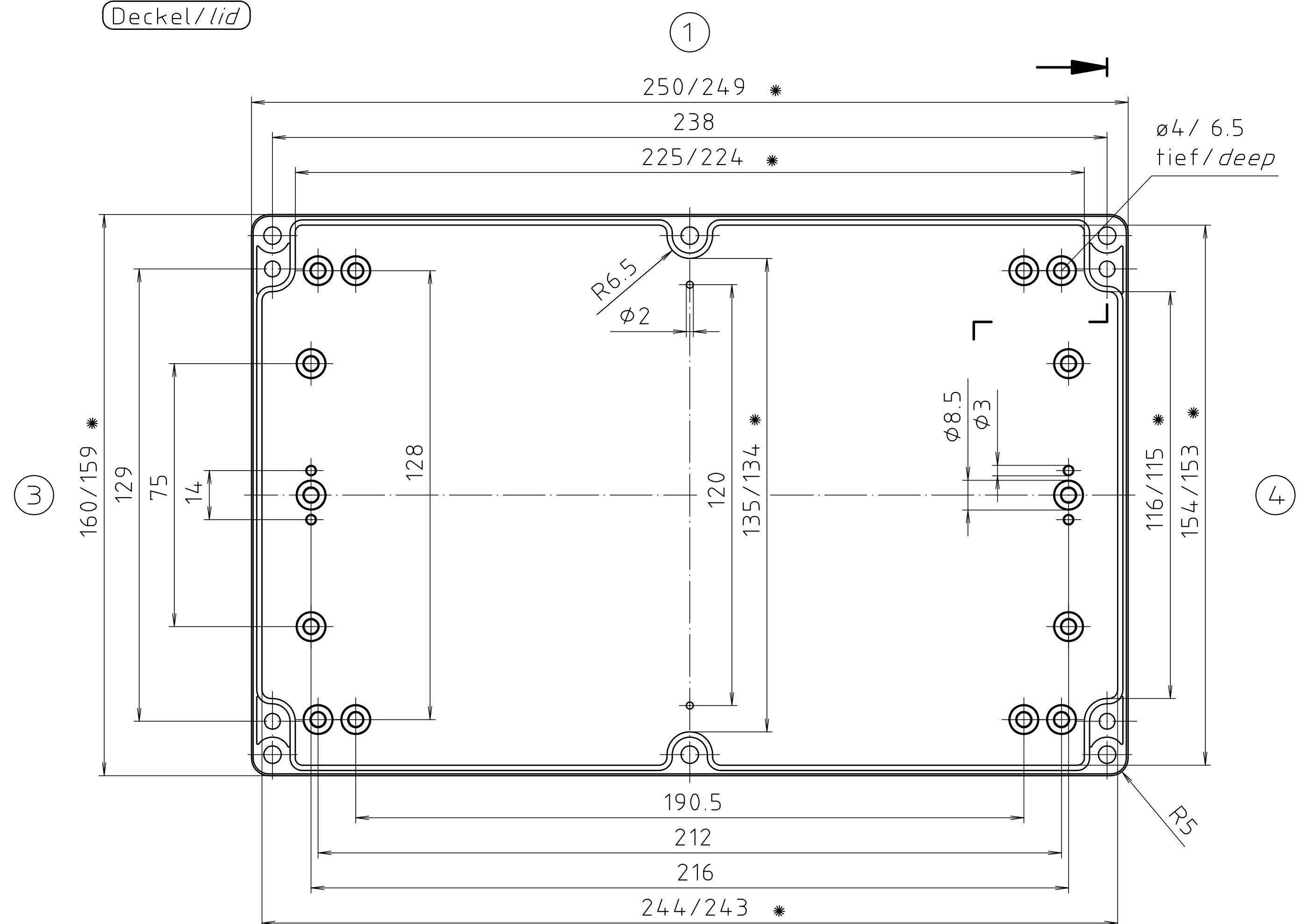
Unterteil/base
