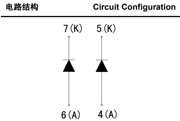
图 1.电路结构
