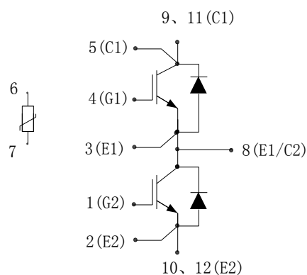
图 1. 电路结构
