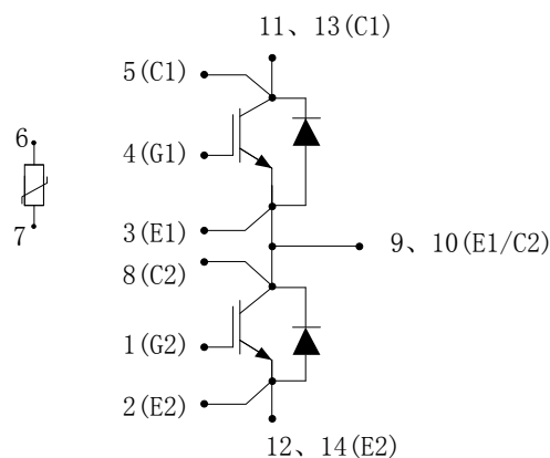
图 1. 电路结构
