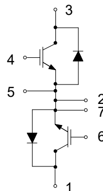
图 1. 电路结构
