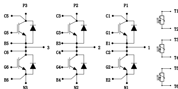
图 1. 电路结构
