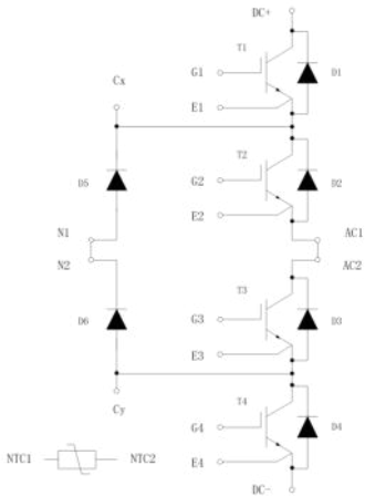
图 1. 电路结构 Fig. 1 Circuit configuration
