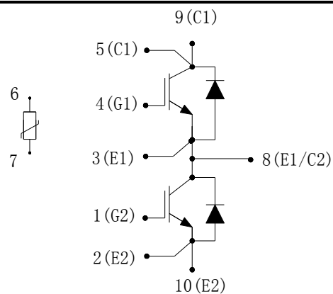
图 1. 电路结构
