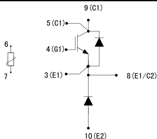
图 1. 电路结构
