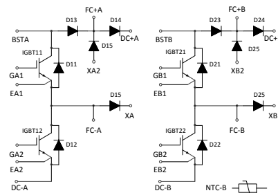
图 1. 电路结构
