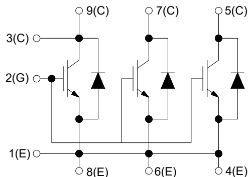
图 1. 电路结构
