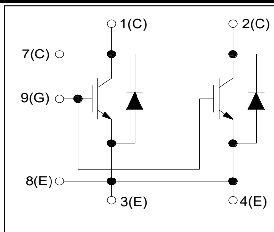
图1. 电路结构
