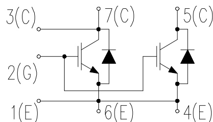
图 1. 电路结构
