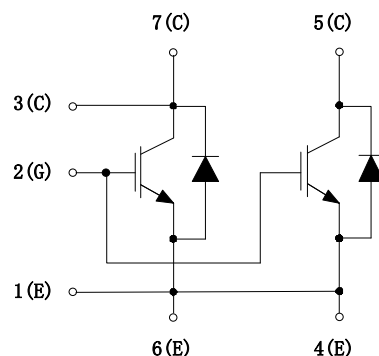
图 1. 电路结构
