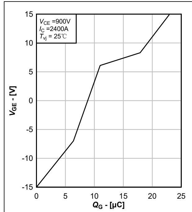
图 16. 栅极电荷特性典型曲线, V_{GE} = f(Q_G)
