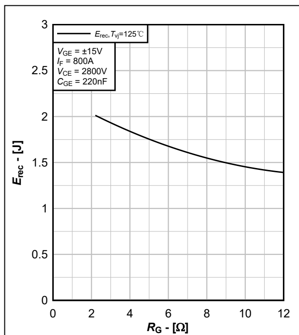
图 13. FRD 反向恢复损耗典型曲线, E_{rec} = f(R_G)
