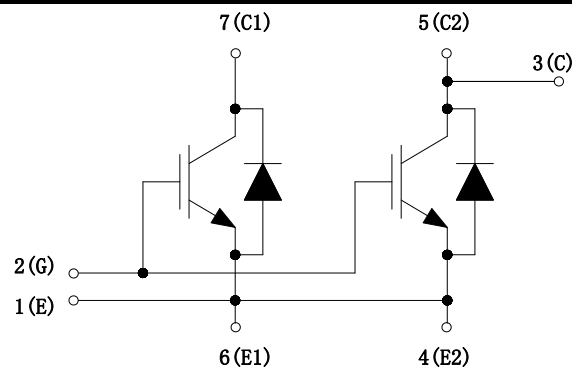
图 1. 电路结构
