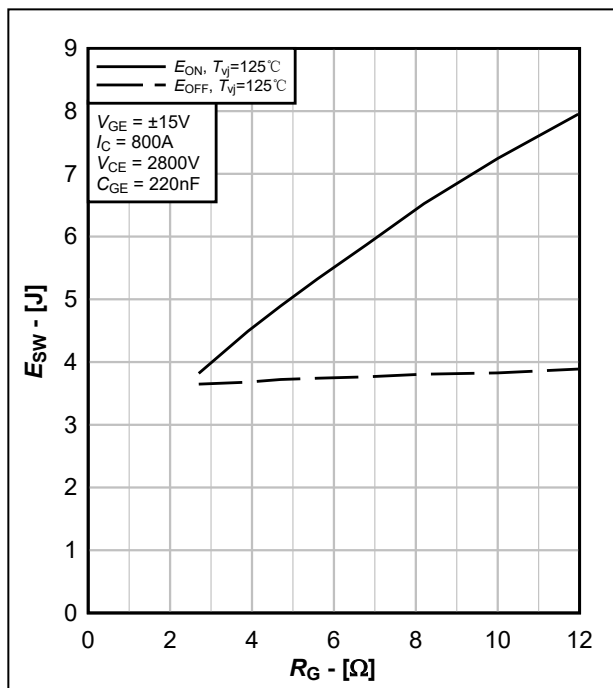
图 7. IGBT 开关损耗典型曲线, E_{on}=f(R_G) , E_{off}=f(R_G)
