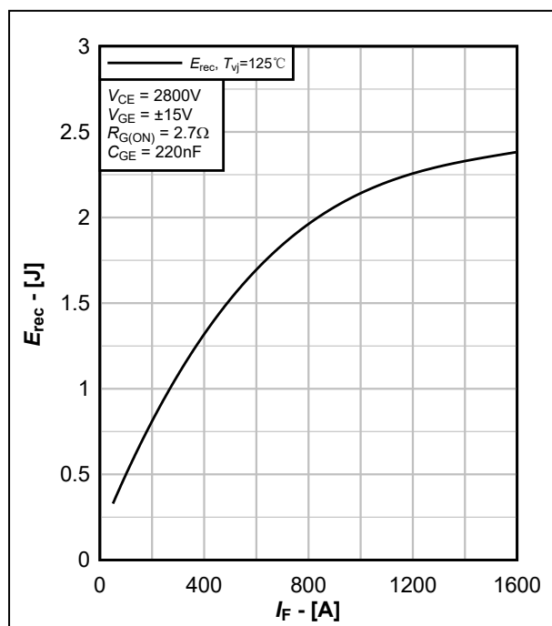
图 12. FRD 反向恢复损耗典型曲线, E_{rec} = f(I_F)
