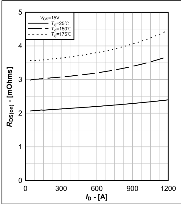
图 7. 导电电阻典型曲线, R_{DS(on)} = f(I_D)
