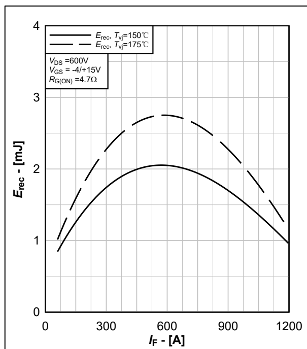
图 14. 体二极管反向恢复损耗典型曲线, E_{rec} = f(I_F)
