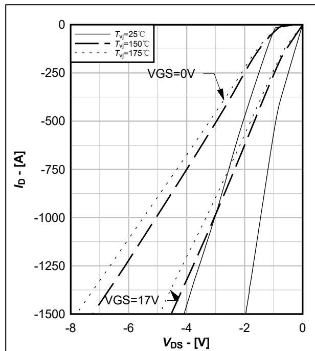
图 11. 体二极管及第三象限输出特性典型曲线, I_D = f(V_{DS})
