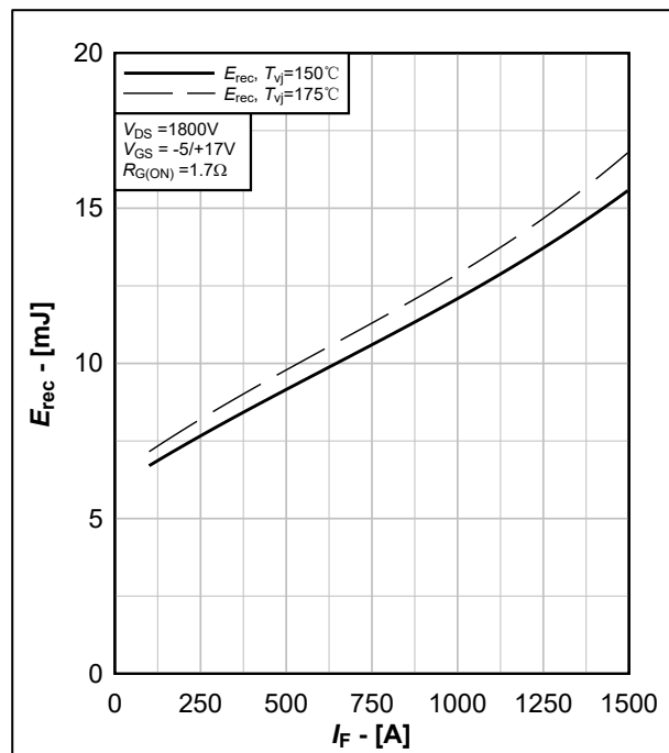
图 12. 体二极管反向恢复损耗典型曲线, E_{rec} = f(I_F)
