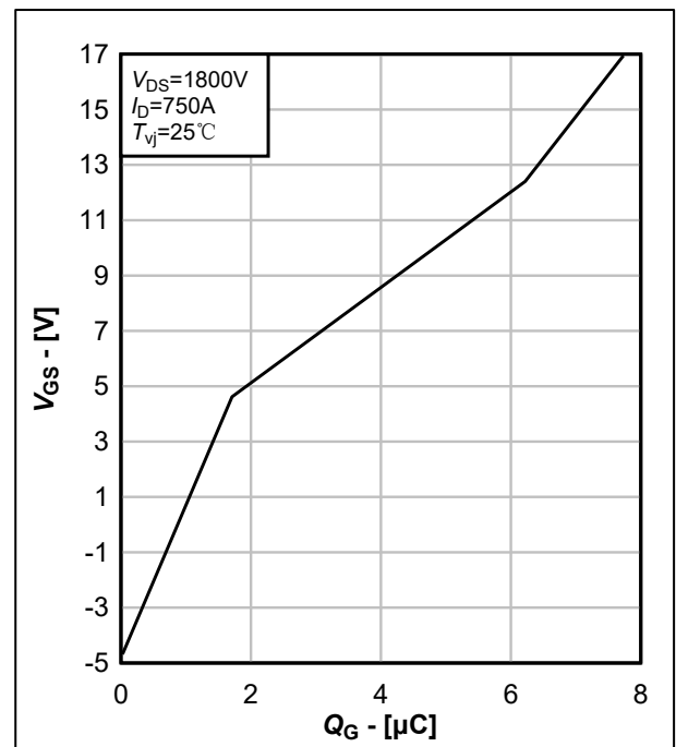
图 10. 栅极电荷特性典型曲线, V_{GS} = f(Q_G)
