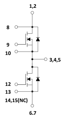
图 1. 电路结构
