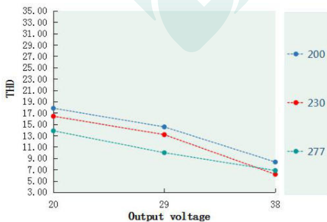
T.H.D. VS Output voltageDL-100I-V38P/A-MAS)
