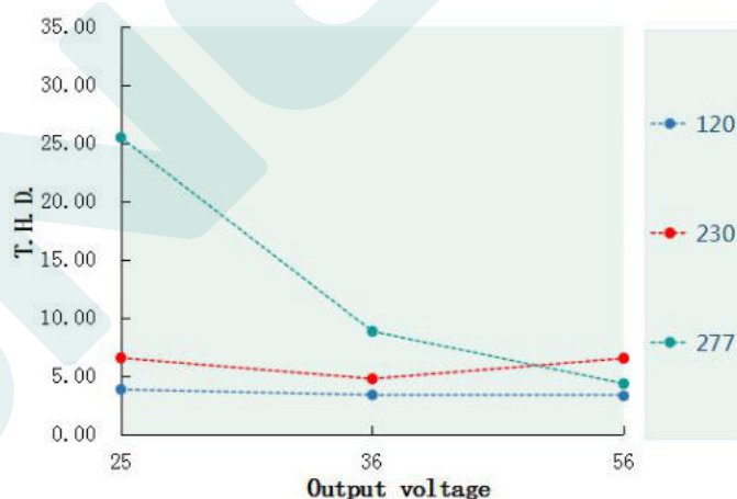
T.H.D. VS Output voltage(DL-100W-V56A/P/X-MDK)
