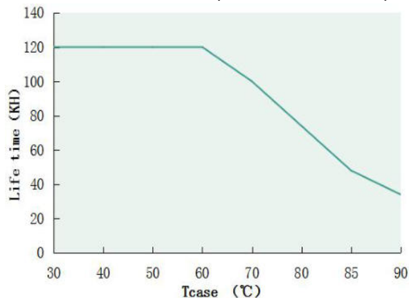
Tcase VS Lifetime (DL-100W-A/P/X-MXG)
