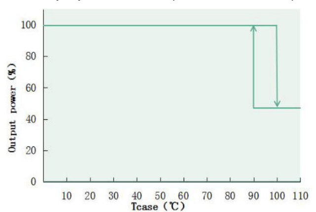
Output power VS Tcase (DL-100W-A/P/X-MXG)
