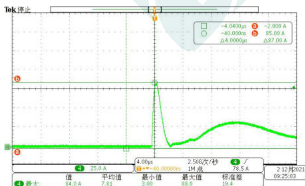
Inrush Current(DL-150H-A/P-MAS)
