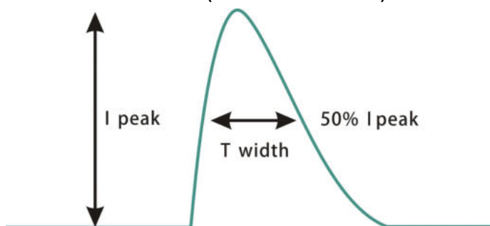
Inrush current(DL-150W-A/P/X-MXG)
