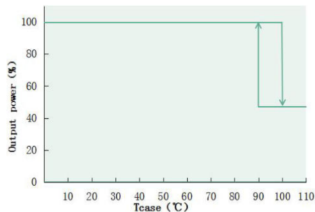
Output power VS Tcase (DL-150W-A/P/X-MXG)
