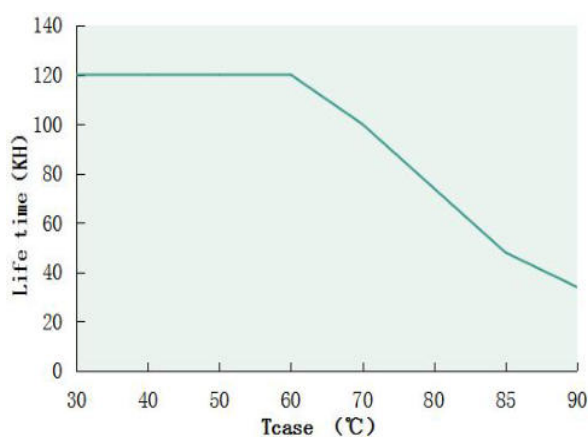
Tcase VS Lifetime(DL-150W-A/P/X-MXG)
