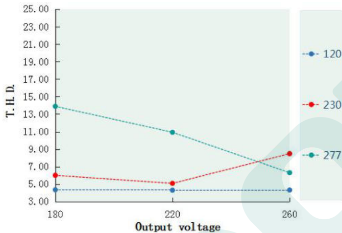
T.H.D. VS Output voltage(DL-150W-V260A/S/X-SPF)
