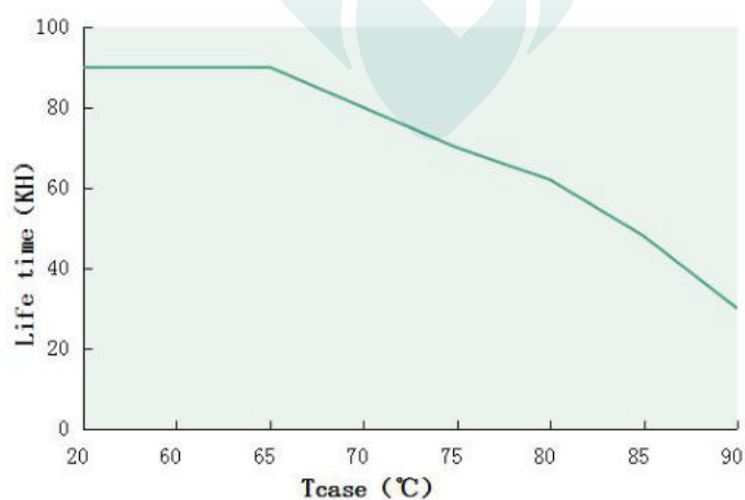
Tcase VS Lifetime(DL-200H-P/X-MXK)
