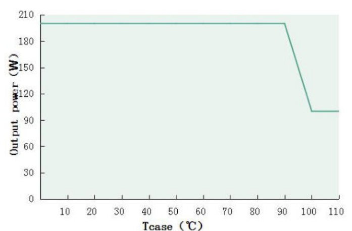
Output power VS Tcase (DL-200H-P/X-MXK)
