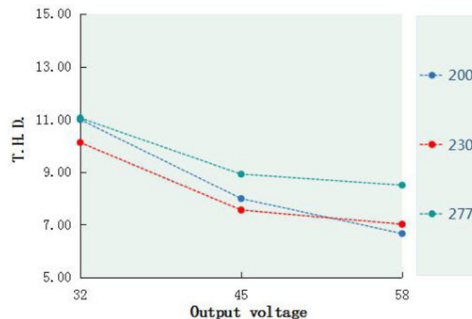
T.H.D. VS Output voltage(DL-200H-V58P/A-MAS)
