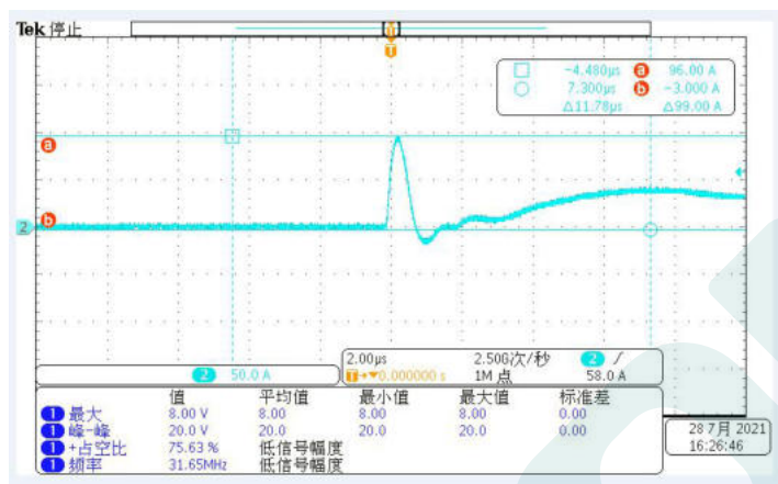
Surge curve(DL-200H-P/A-MAS)
