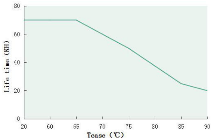
Tcase VS Life time(DL-200H-P/A-MAS)
