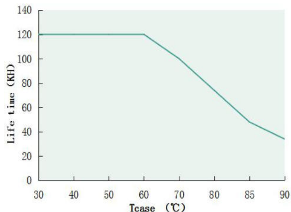
Tcase VS Lifetime(DL-200W-A/P/X-MXG)
