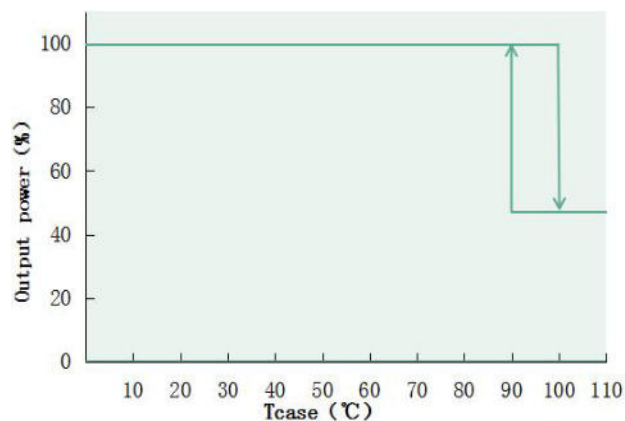
Output power VS Tcase (DL-200W-A/P/X-MXG)
