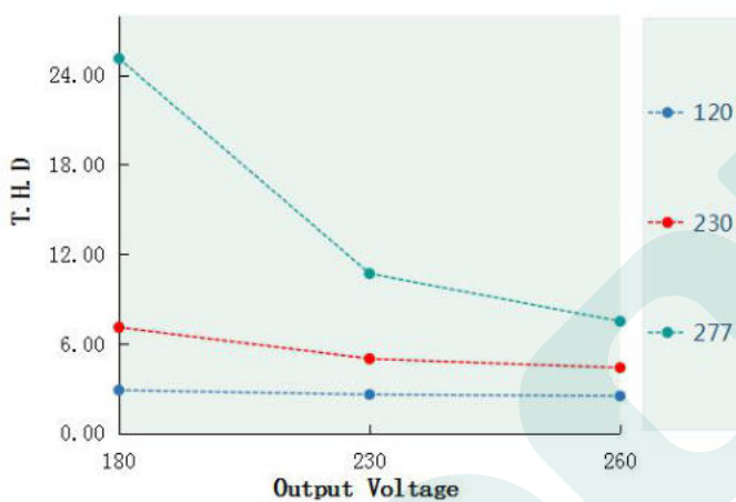
T.H.D. VS Output voltage (DL-200W-V260A/S/X -SPF)
