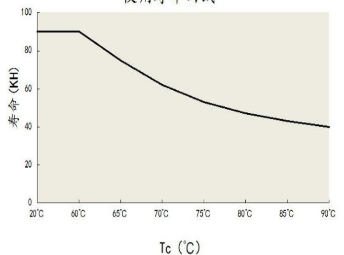
使用寿命曲线
