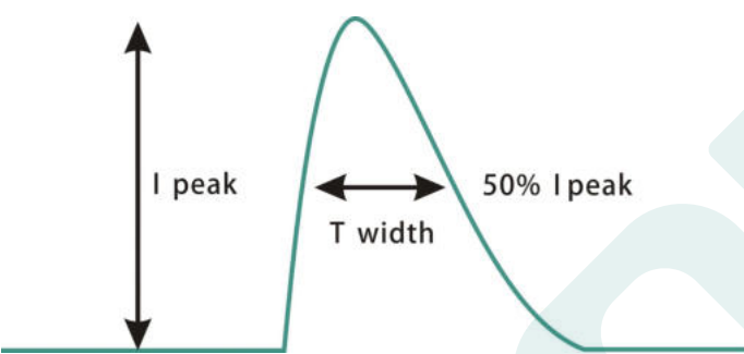
Inrush Current(DL-240H-A/P-MAS)
