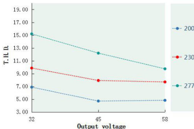
T.H.D. VS Output voltage(DL-240H-V58P/A-MAS)
