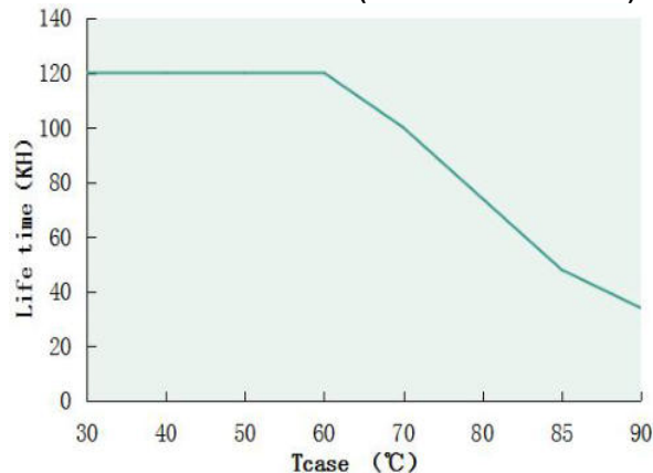
Tcase VS Lifetime(DL-240W-A/P/X-MXG)
