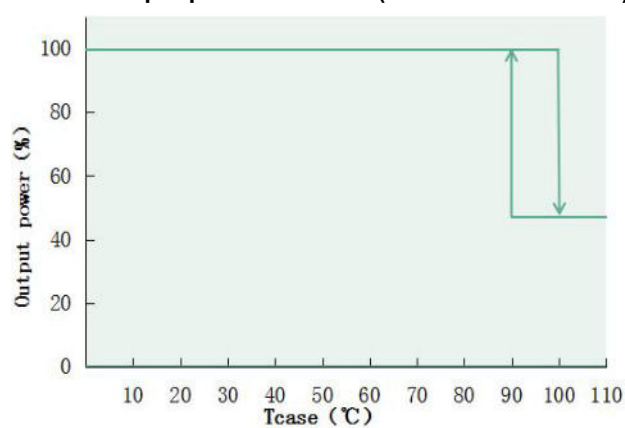
Output power VS Tcase (DL-240W-A/P/X-MXG)
