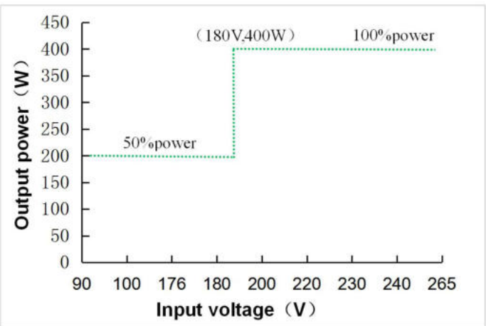
Output power VS Input voltage(V24 V36 V48)
