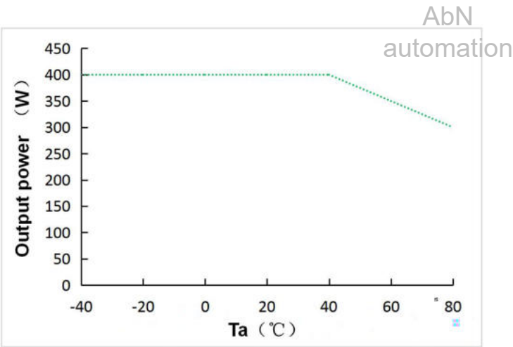
Output power VS Ta (V24 V36 V48)
