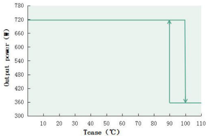
Output power VS Tcase (DL-720W-MXG)
