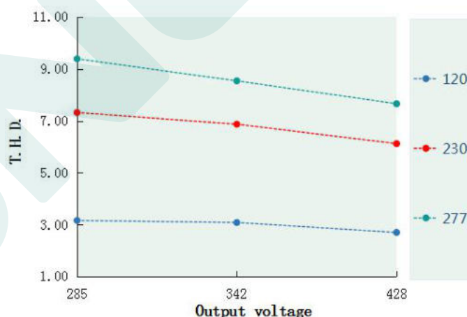
T.H.D. VS Output voltage(DL-720W-V428X/T-MXG)
