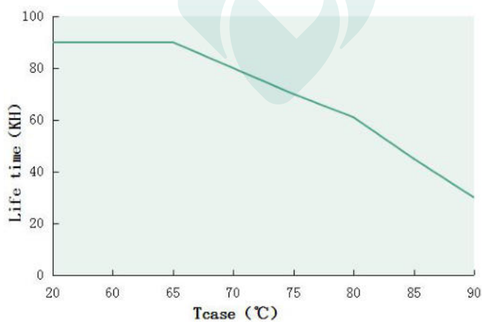
Tcase VS Lifetime(DL-75W-A/P/X-MDK)
