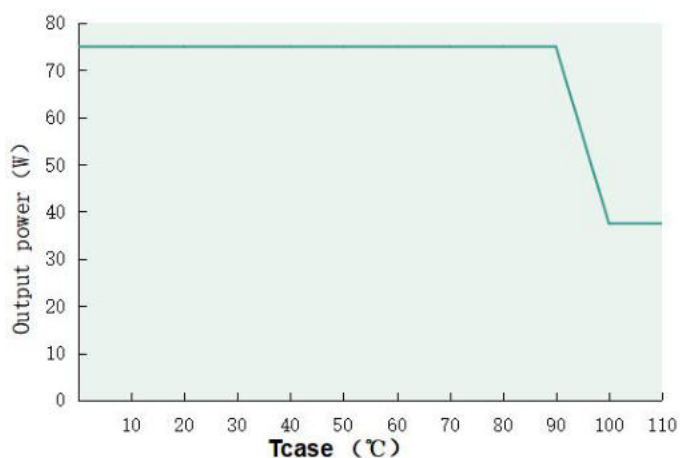
Output power VS Tcase (DL-75W-A/P/X-MDK)
