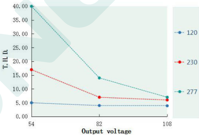
T.H.D. VS Output voltage(DL-75W-V108A/P/X-MDK)
