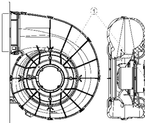
Fig. 1: Installed fan
