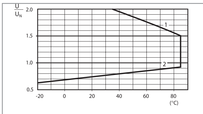
R 40 - Отношение рабочего диапазона для пост. тока к температуре окр. среды. Стандартная обмотка
