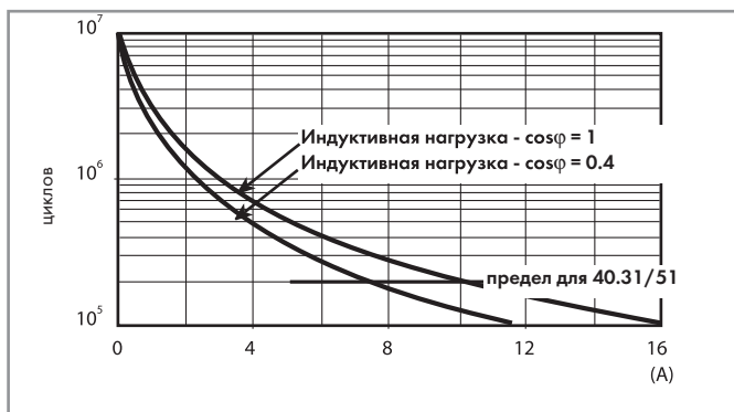
F 40 - Электрическая долговечность (АС) при ном. нагрузке Типы 40.31/51/61
