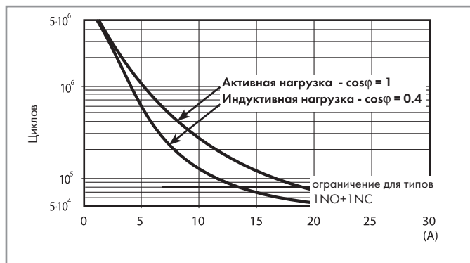
F 65 - Электрическая долговечность (AC) при номинальной нагрузке
