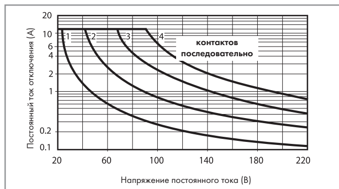
H 56 - Макс. отключающая способность DC1
