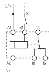
Схема электрических соединений (с сигналом START)
