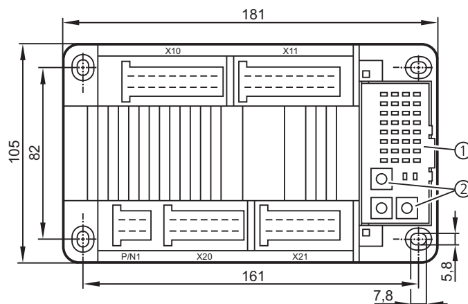
1) LEDs 2) Drehschalter
