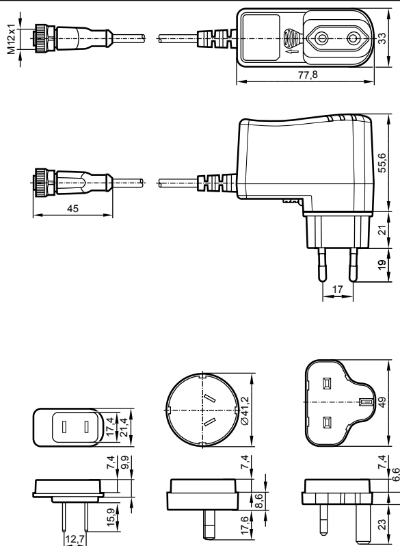
La figure montre l'alimentation débrochable avec adaptateur secteur UE enfilé
