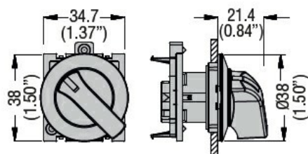
Long lever
