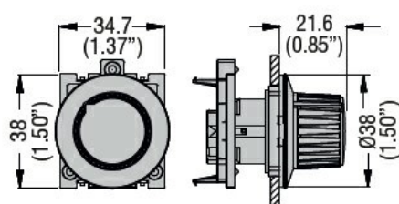
Knob
