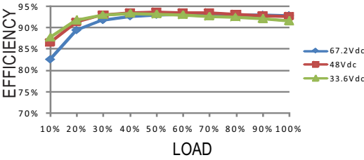
DDR-240C-24
