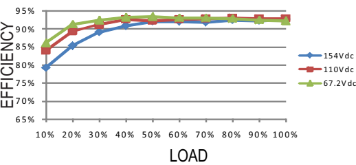
DDR-240D-24
