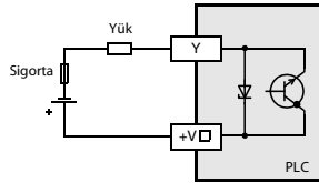
Transistör çıkışı (pozitif)
