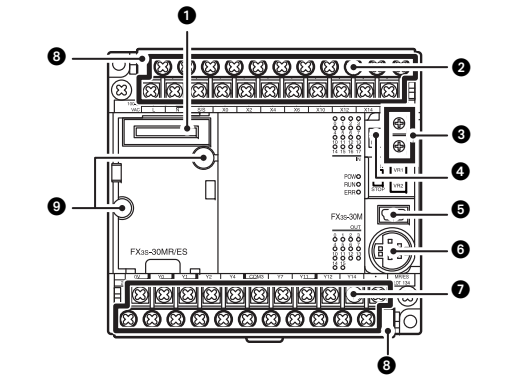
Vue avec les capots déposés
