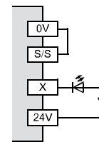
Plusschaltend (Source)
