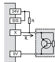
Minuschaltend (Sink)
