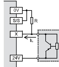
переключение на плюс (Source)
