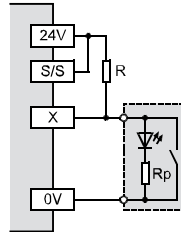
переключение на минус (Sink)
