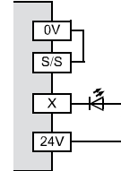
переключение на плюс (Source)
