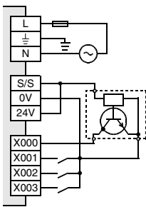
À commutation négative (Sink)
