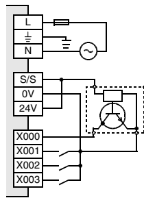
Minuschaltende Geber
