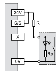
Minuschaltend (Sink)
