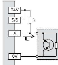
переключение на минус (Sink)
