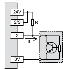
Circuito a logica negativa NPN (Sink)
