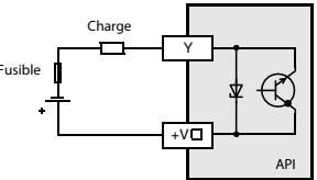
Sortie à transistor (à commutation positive)
