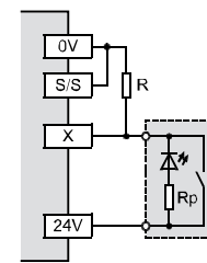
À commutation positive (Source)
