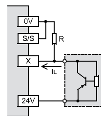
Plusschaltend (Source)
