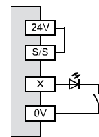
Minuschaltend (Sink)
