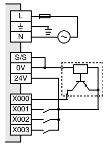
Plusschaltende Geber
