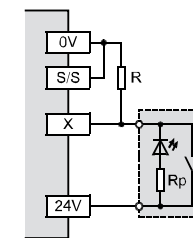
Plusschaltend (Source)
