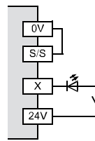
À commutation positive (Source)
