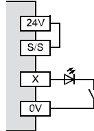
переключение на минус (Sink)
