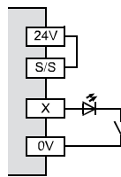
Circuito a logica negativa NPN (Sink)
