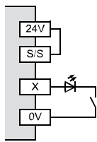
À commutation négative (Sink)
