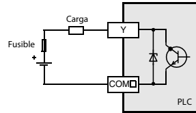
Salida de transistor (NPN)
