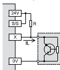
À commutation négative (Sink)
