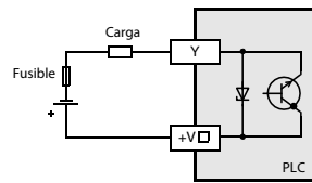
Salida de transistor (PNP)
