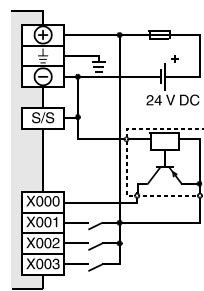
À commutation positive (Source)
