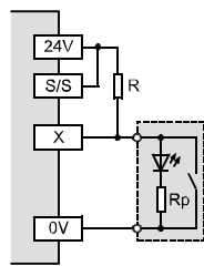
Circuito a logica negativa NPN (Sink)
